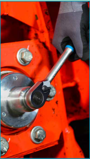
Uruchomienie za pomocą grzechotki poprzez wprowadzony uchwyt 4-kątny 12,5 mm (1/2")
